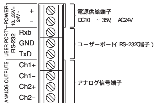
2) 信号と電源供給の配線
