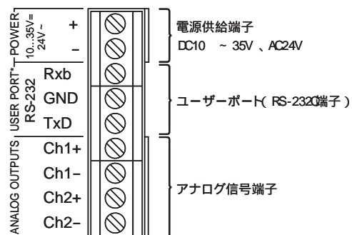
2)信号と電源供給の配線
