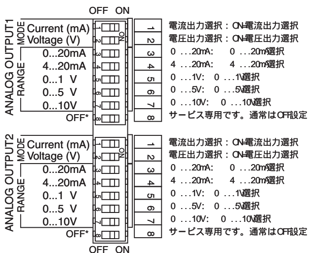
1) アナログディップスイッチ配置図
