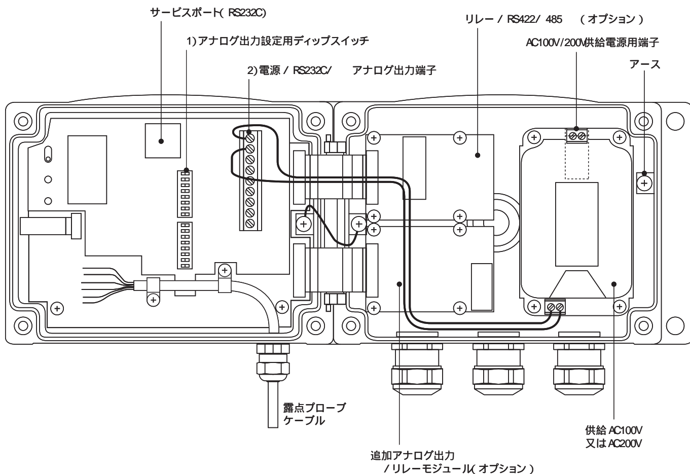
1) アナログディップスイッチ配置図
